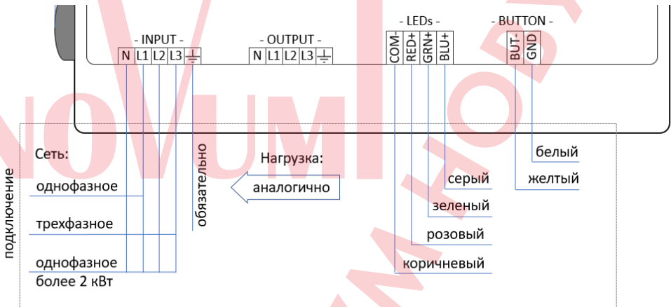
Рис. 1. Схема подключения (подробнее см. п. 4 стр. 5):
